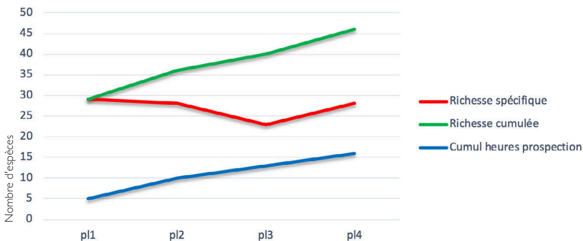
Figure 4 : Cros de Cagne : richesse spécifique
